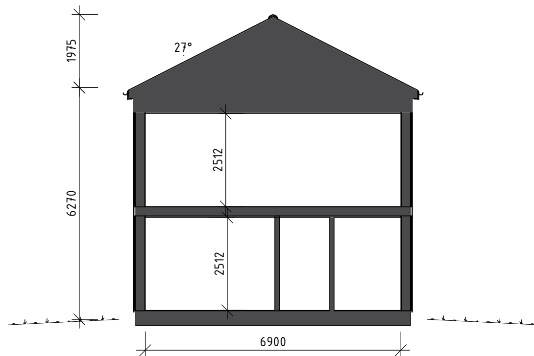
SEKTION A-A
