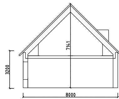
SEKTION A-A
