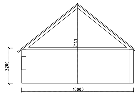
SEKTION B-B
